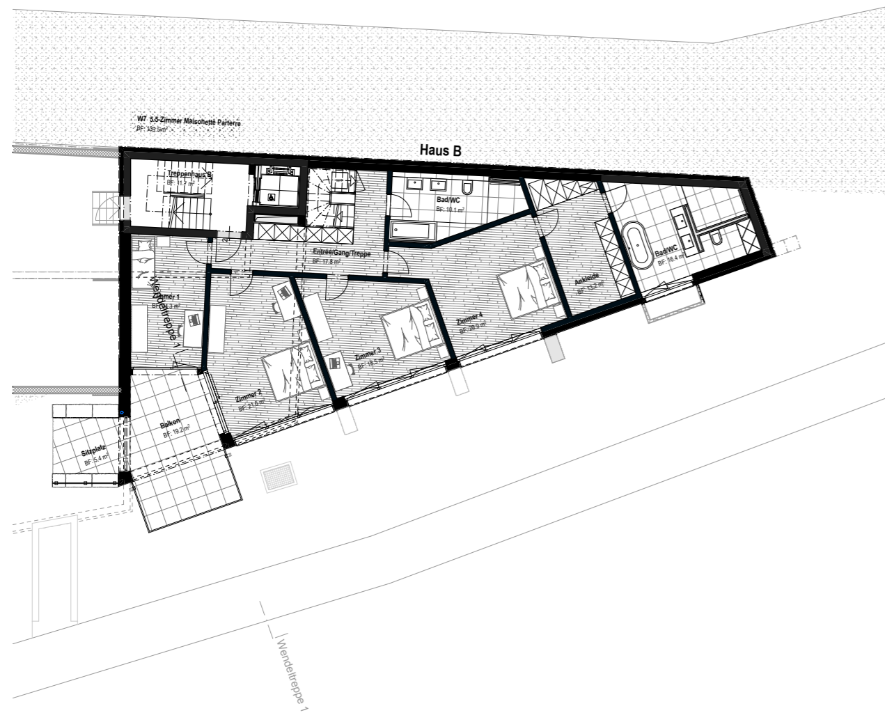
Sockelgeschoss
