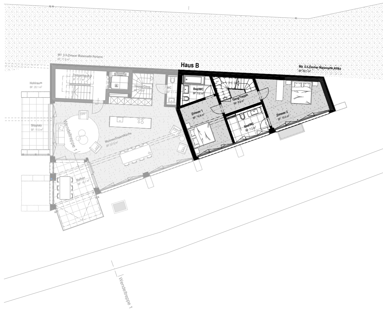
Erdgeschoss
